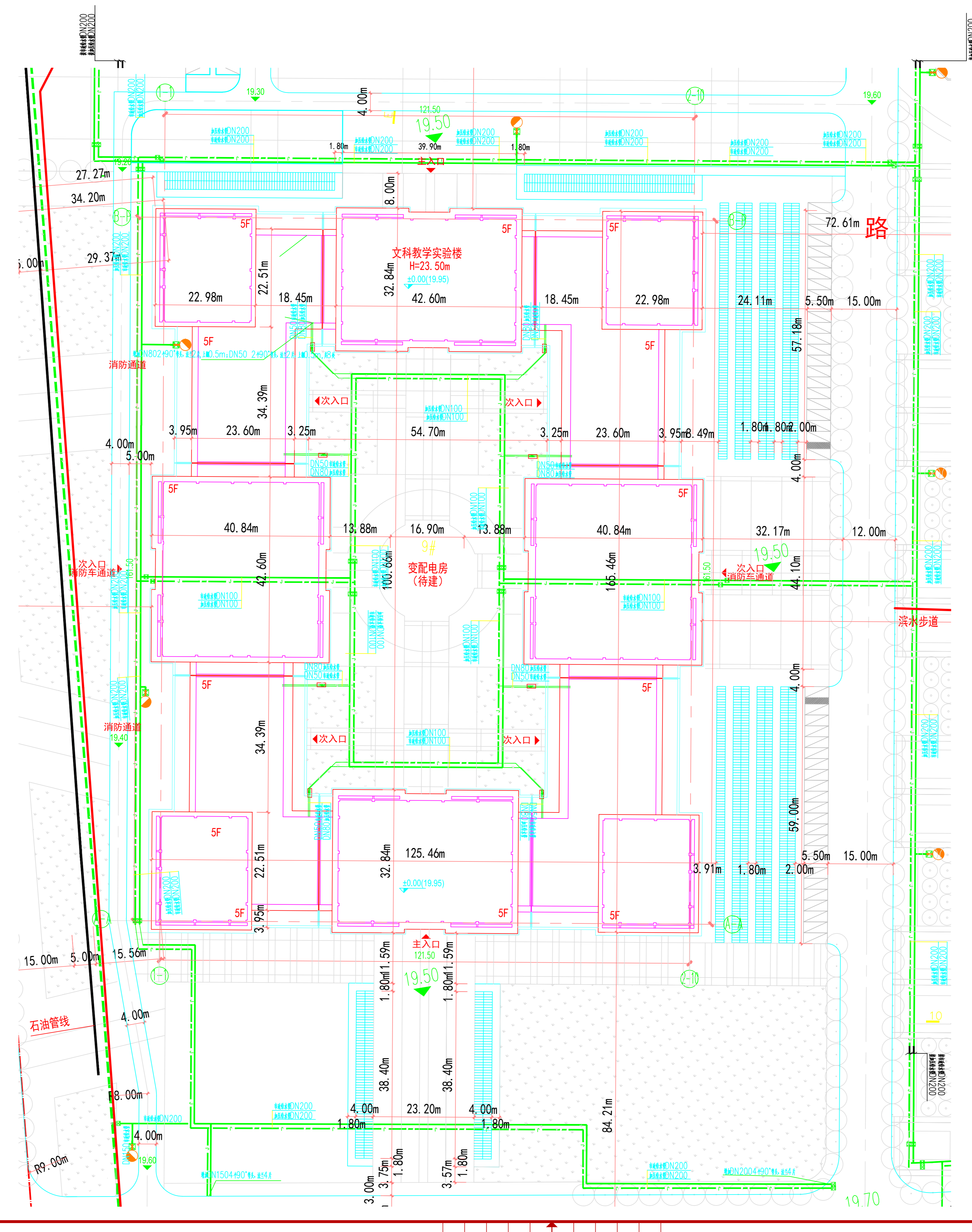
给水总平面图 1:500
