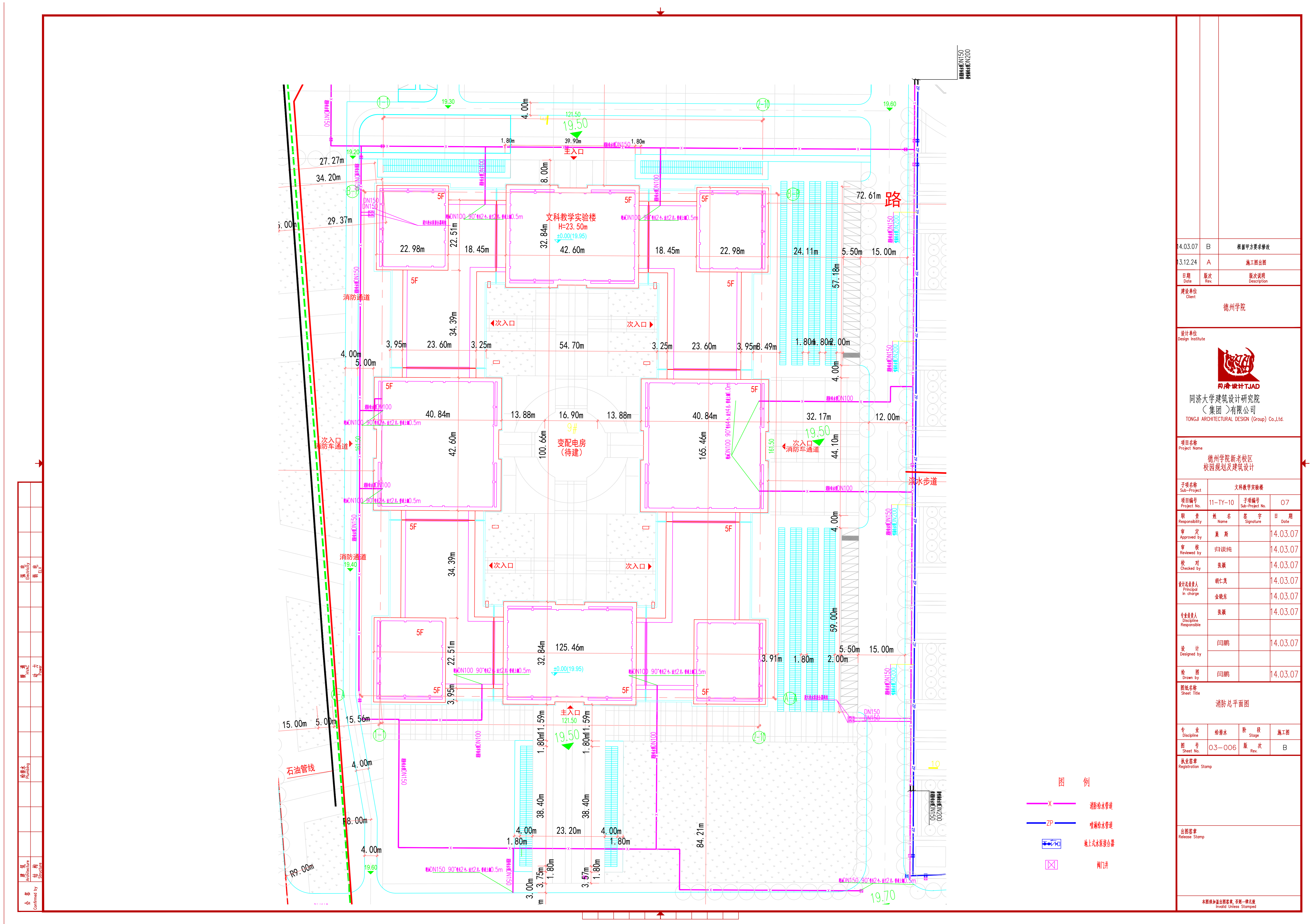
消防总平面图 1:500
