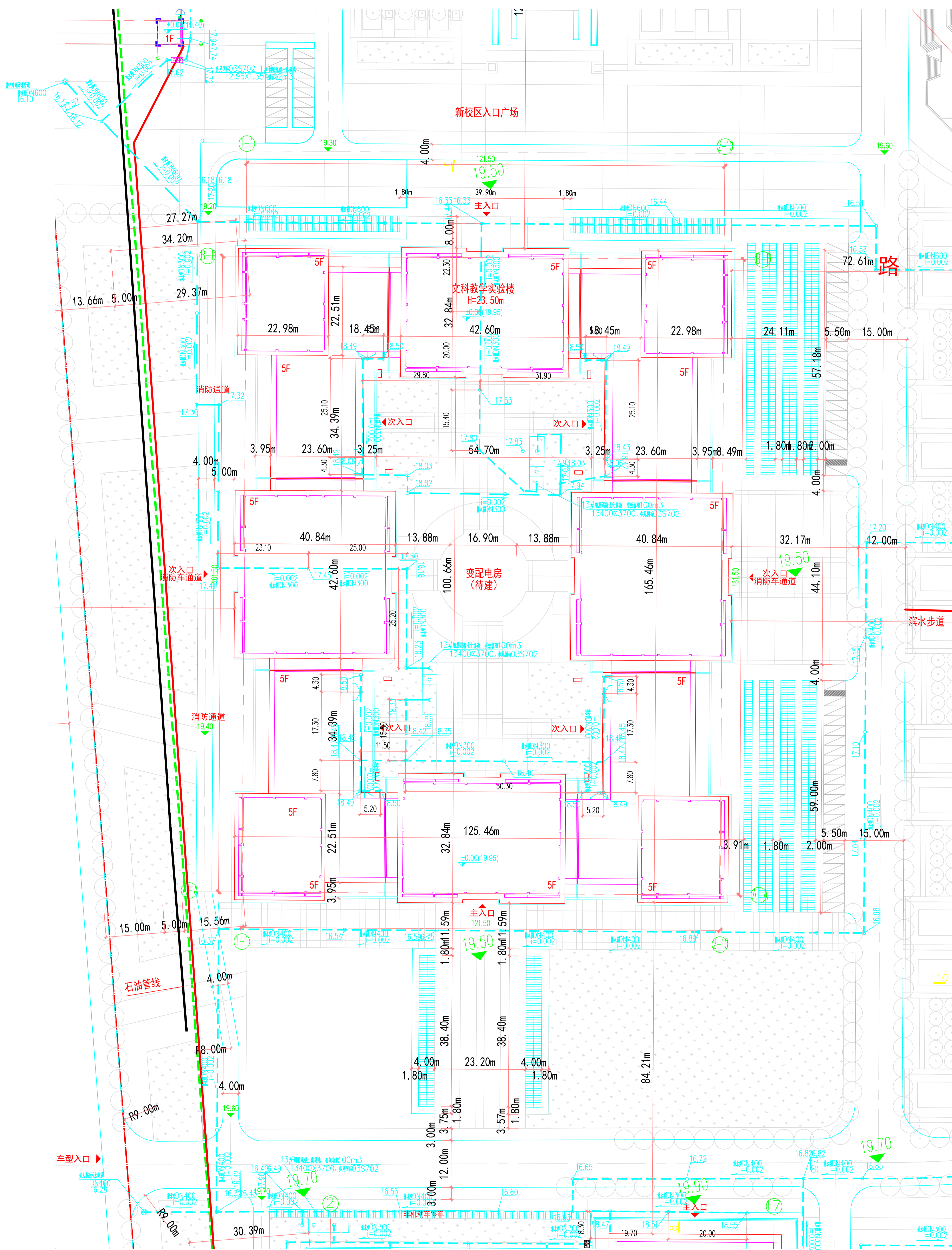
排水总平面图 1:500
